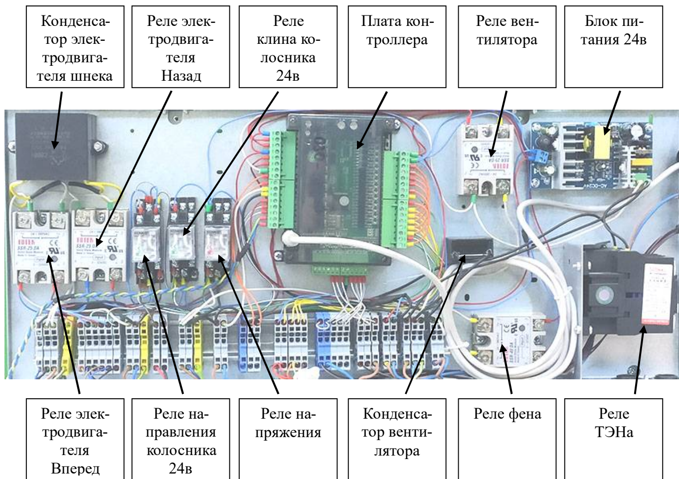
Рис. 1 - Устройство котла О30
