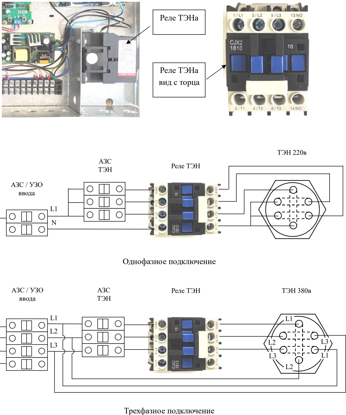
Рис. 6 - Подключение ТЭН
