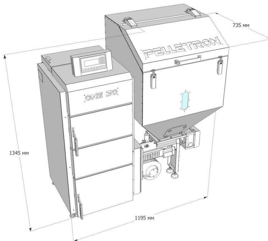
Рис. 2 - Габаритные размеры котла О30
